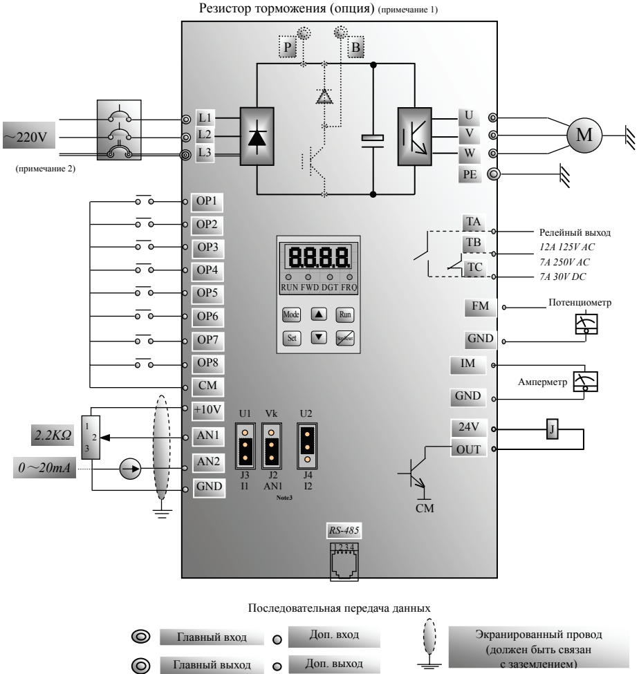
Рис 3-3 Стандартная схема подключения однофазного ПЧ
