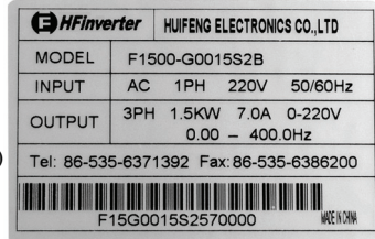
Рис 2-2 Информационный шильдик
