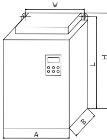
Рис 3-2 Размеры преобразователя F1500-G
