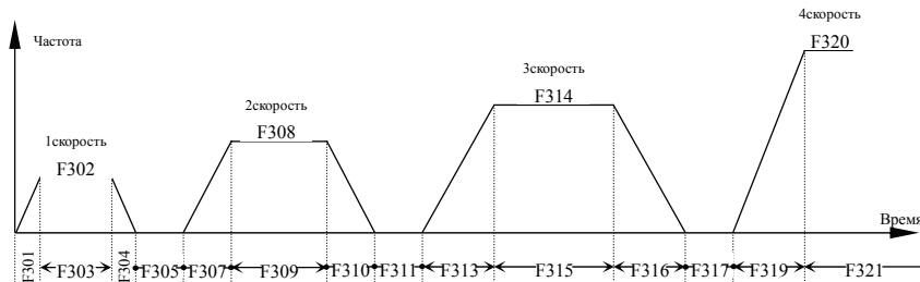
Рис 6-3 Переход к следующей частоте после ожидания
