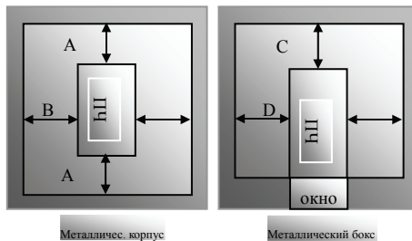
Рис 3-1 Установочные размеры
