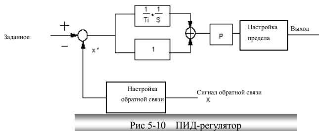
Рис 5-10 ПИД-регулятор
