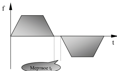
Рис 5-1 Мертвое время переключения
