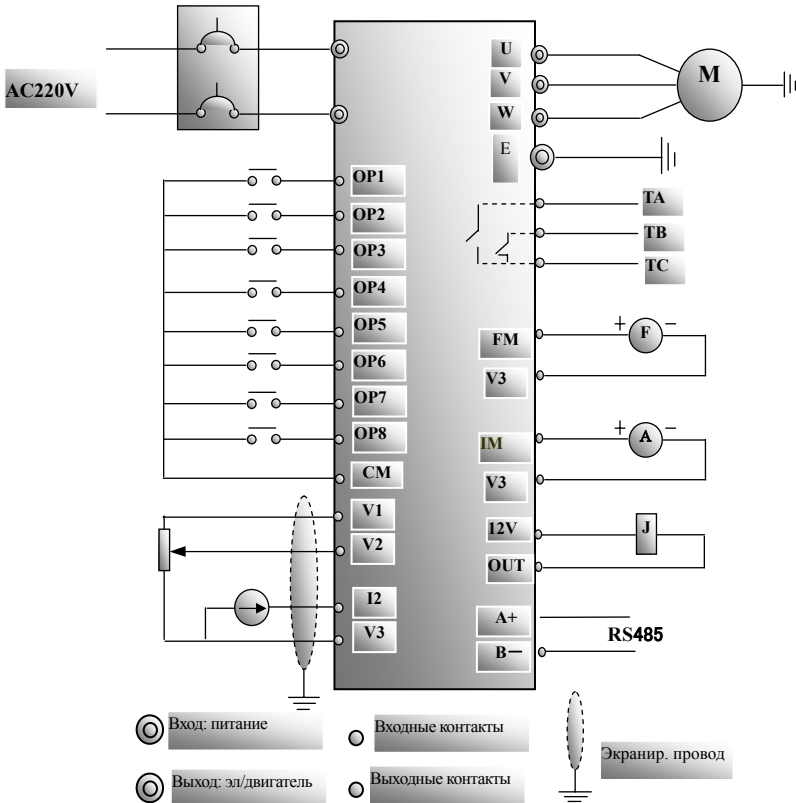
Рис.3-2 Схема подключения однофазного преобразователя
