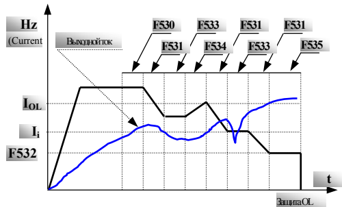
Рис.9-3 Настройка торможения
